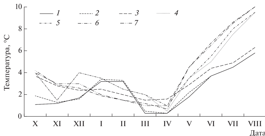
Рис. 2. Годовой ход минимальных месячных температур в местах зимовки Ranodon sibiricus в долине р. Борохудзир по данным логгеров. Местоположение логгеров см. на рис. 1а–1в и в тексте.
